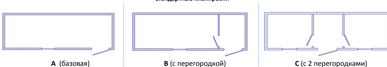
Стандартные планировки
